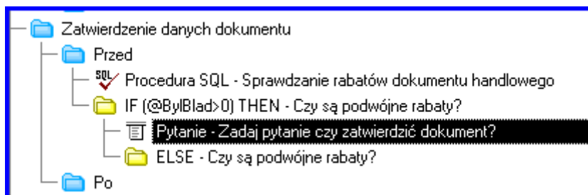
Rys. 21 Stan gniazda po przeniesieniu Pytania (Przykład 2)
