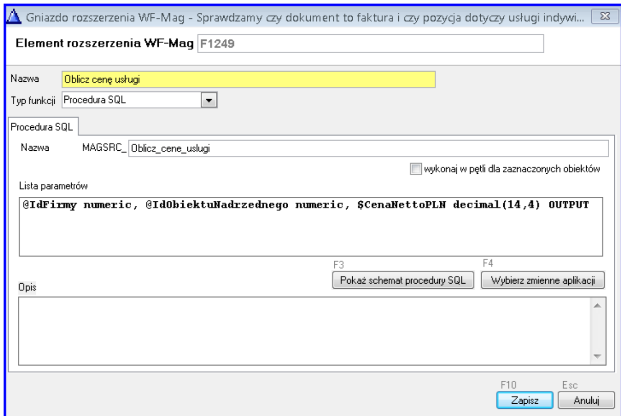
Rys. 39 Definicja procedury obliczenia ceny usługi (Przykład 4)
